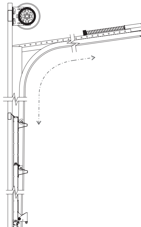
Fig. 2- Detalle de puerta con guías inclinadas.
